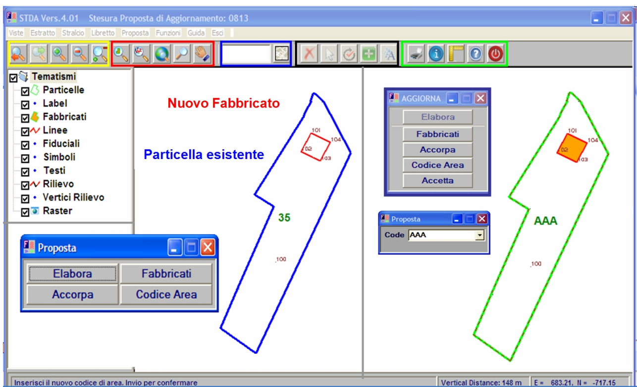
Fig. 1 - Nuova interfaccia grafica implementata nella procedura Pregeo 10 ed esemplificazione della predisposizione della proposta di aggiornamento cartografico.
